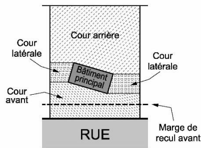
Croquis 2.6 Localisation des cours pour un bâtiment
